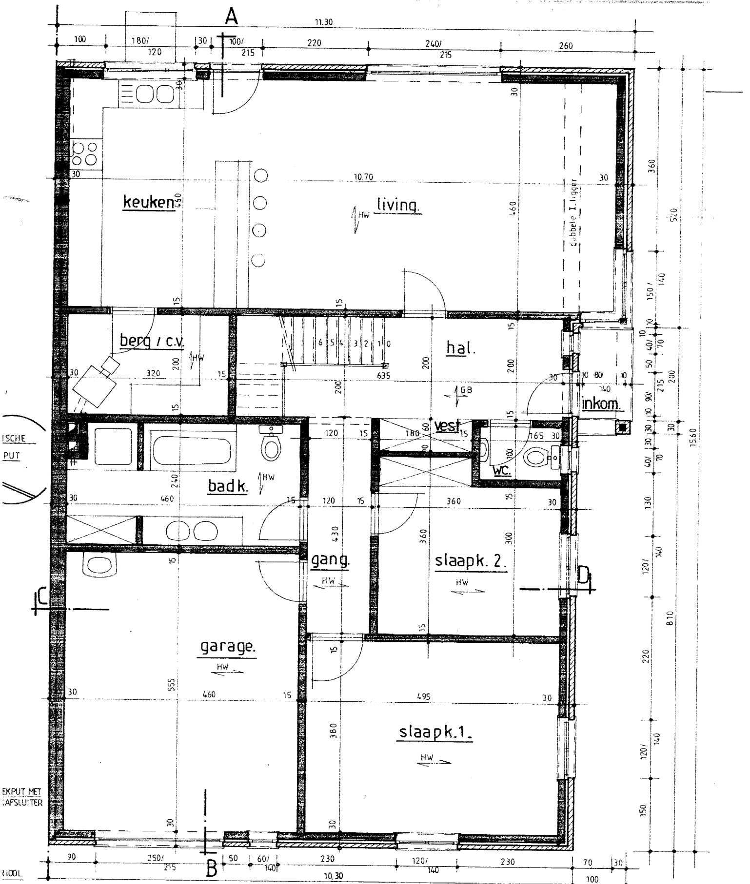
GRONDPLAN.
